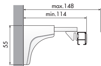
art. P4142 Fissaggio a parete
