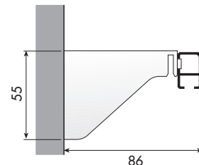
art. P4085 Fissaggio a parete
