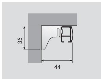
art. P4083 Fissaggio a parete
