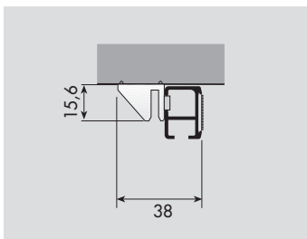
art. P4081 Fissaggio a soffitto
