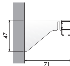
art. P4084 Fissaggio a parete
